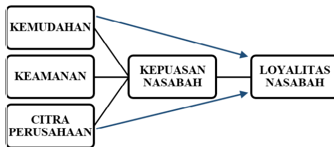
Gambar 3.1 Uji Sobel
